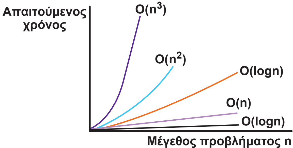
Εικόνα 2.10: Καμπύλες των κυριότερων συναρτήσεων πολυπλοκότητας.
