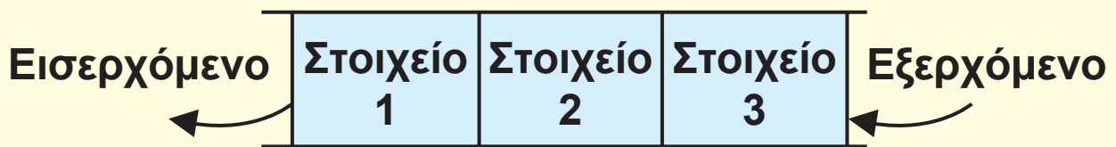
Εικόνα 2.15. Ουρά
