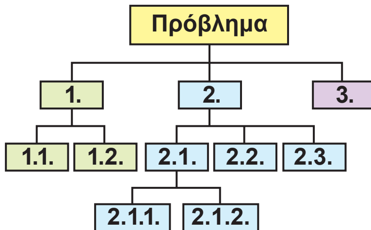
Εικόνα 2.5.
