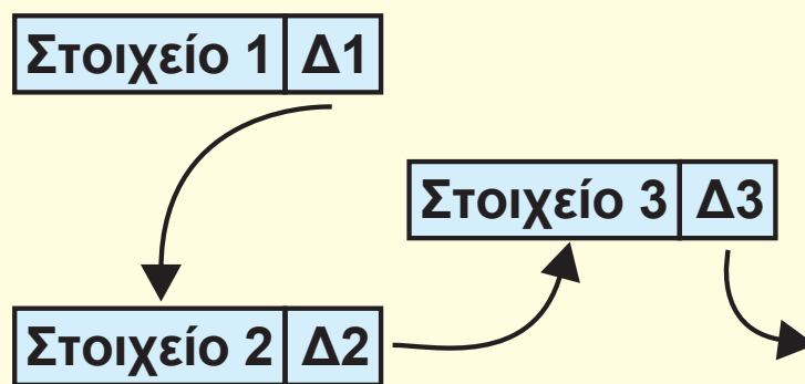
Εικόνα 2.16. Λίστα
