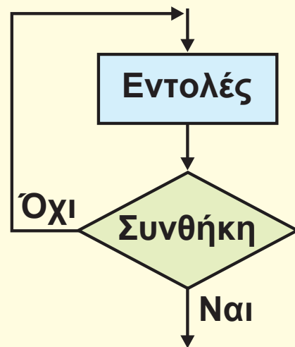
Εικόνα 2.23.
