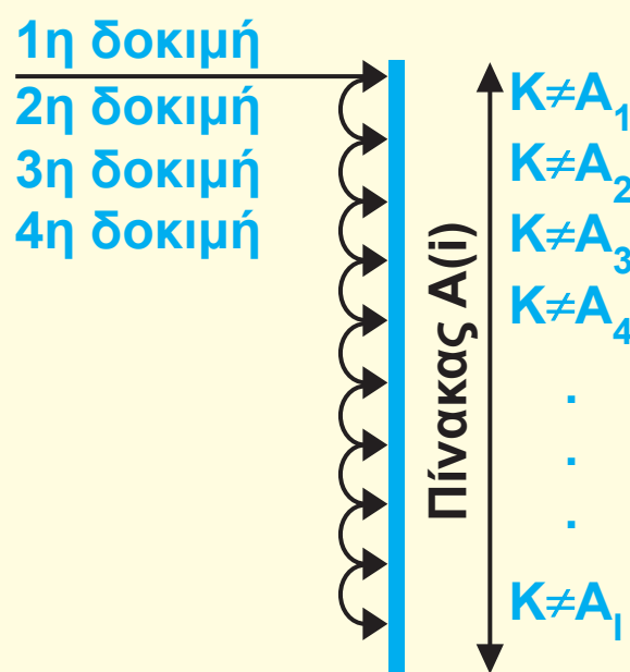
Εικόνα 2.24. Σειριακή αναζήτηση.
