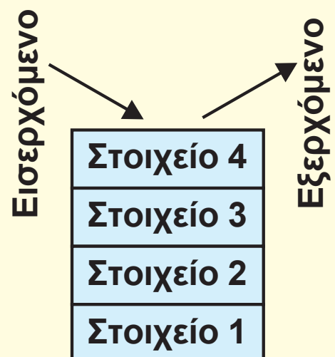
Εικόνα 2.14. Στοιίβα
