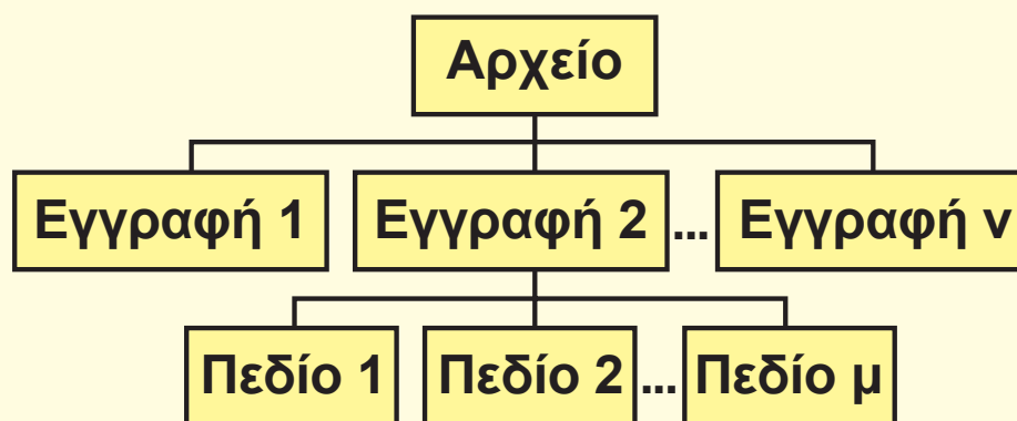
Εικόνα 2.19. Δομή αρχείου
