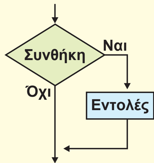
Εικόνα 2.20.
