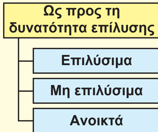
Εικόνα 2.2. Κατηγορίες προβλημάτων
