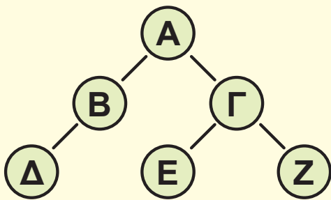
Εικόνα 2.17. Δένδρο
